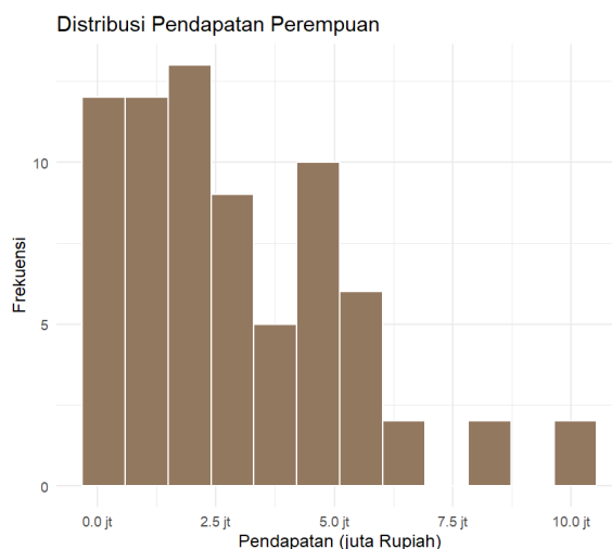
Gambar 4. Distribusi Pendapatan Perempuan
